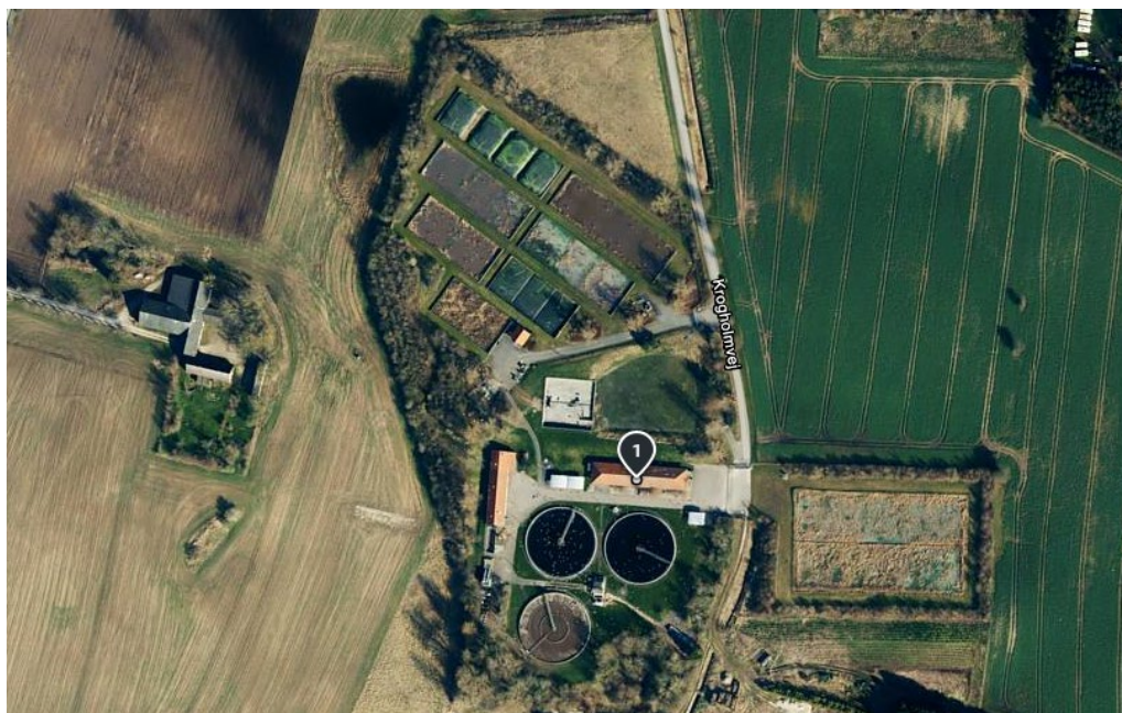
Figur 4 Jyllinge Renseanlæg
