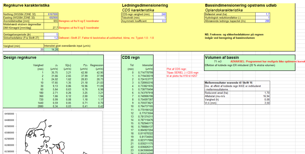
Figur 2 Eksempel med erhverv med lokal forsinkelse og afledning til ny offentlig kloak
