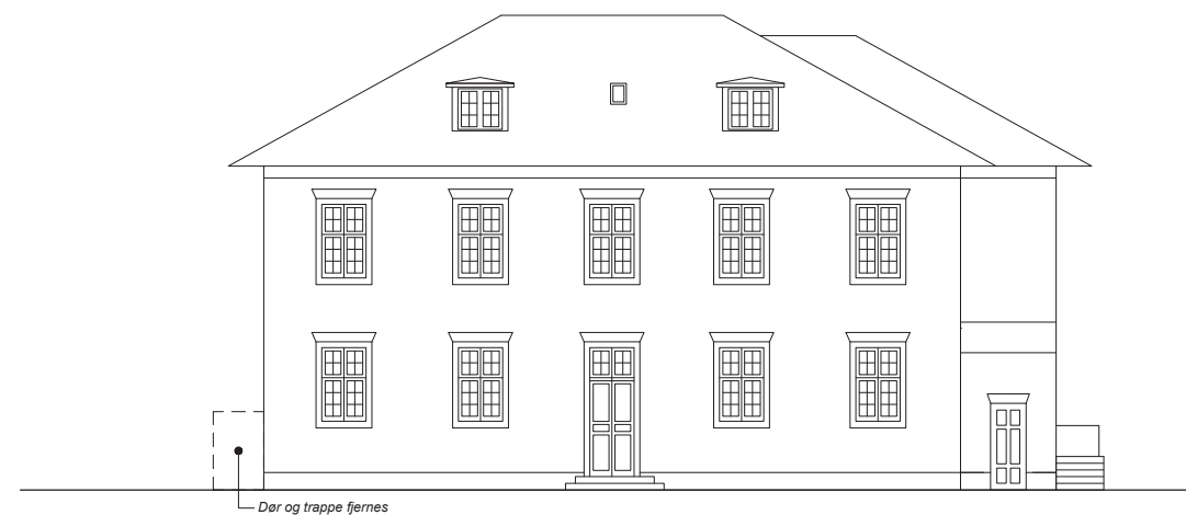
Fremtidig østfacade
