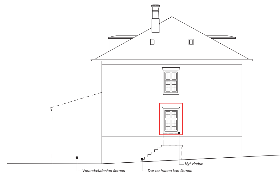
Fremtidig sydfacade
